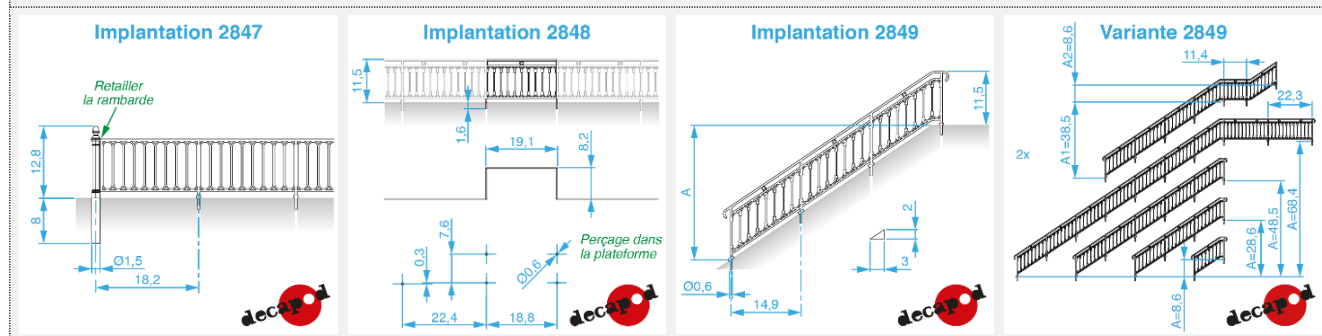
Mise en oeuvre rambardes type Creil-Beauvais réf 2841 Réseau Epoque III, Eric Goasdoue. Meursault 2013
